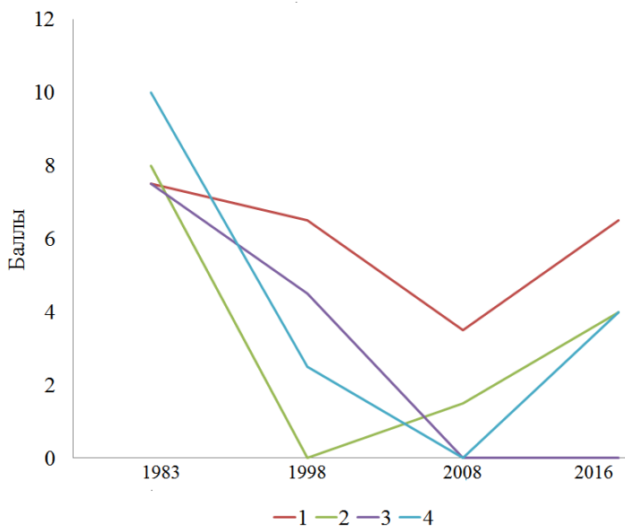
Рисунок 14 – Изменение интегральной оценки по годам в подводных ландшафтах бухты Ласпи.
